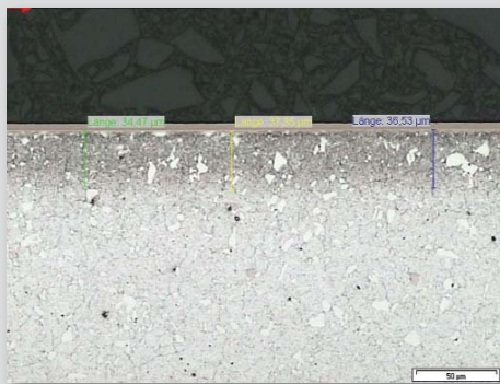
Sección transversal con capa de difusión
