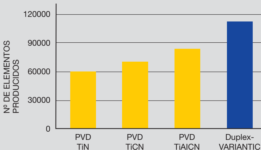
Matriz de conformación D2, recubrimiento Duplex-VARIANTIC; material de trabajo: acero 1.0335 laminado en caliente.
